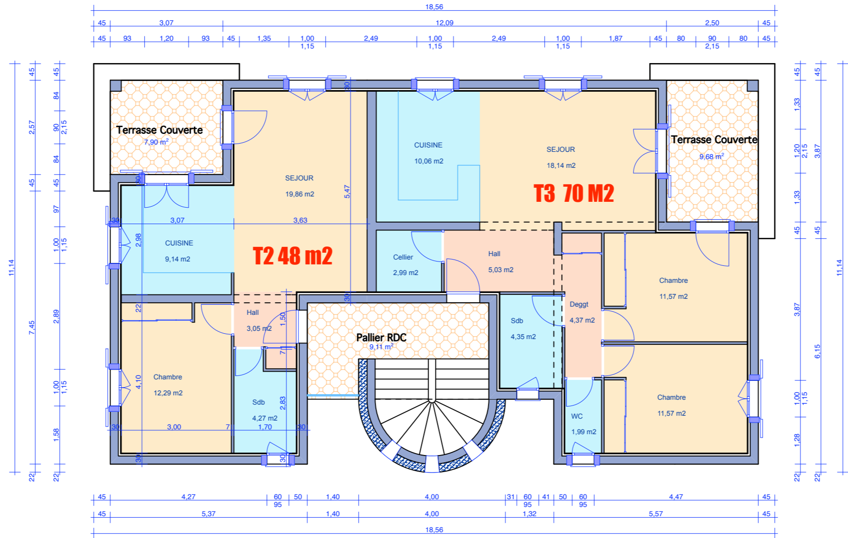
PLAN NIVEAU R+1 ECHELLE 1/100
